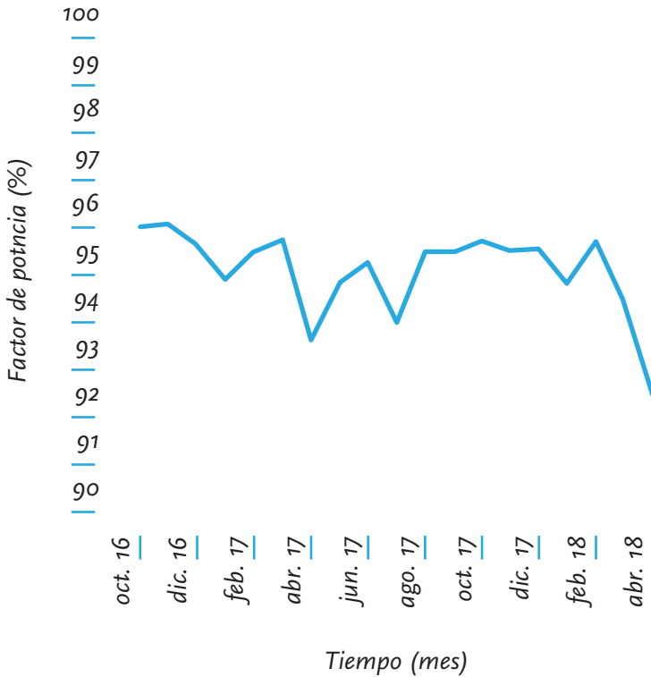
Gráfica 3. Análisis del comportamiento de la relación tiempo-factor de potencia, en el edificio “K” en la Universidad Tecnológica de San Juan del Río.
