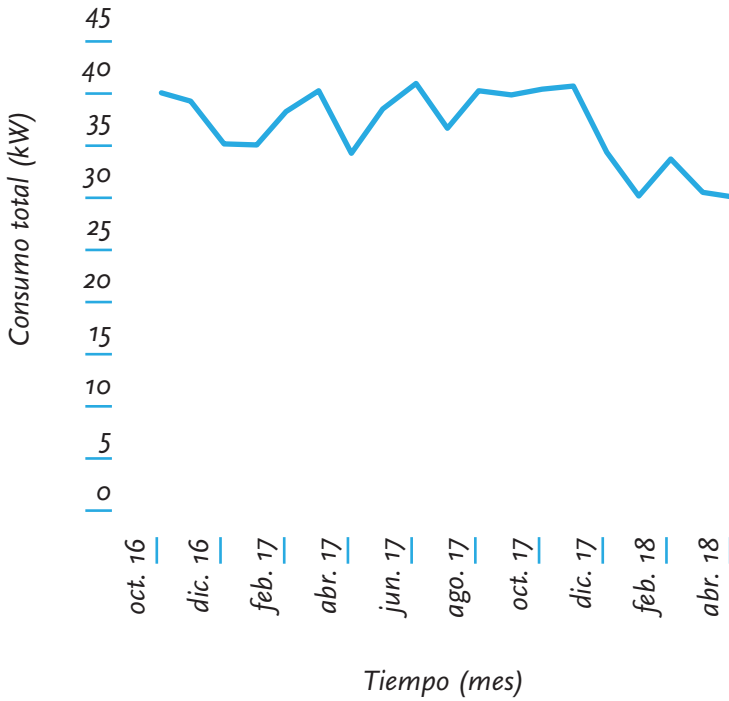
Gráfica 2. Análisis del comportamiento de la relación tiempo-consumo total kWh, en en el edificio “K” en la Universidad Tecnológica de San Juan del Río.
