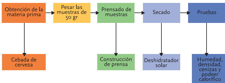
Figura 5. Proceso de elaboración de Briquetas.
