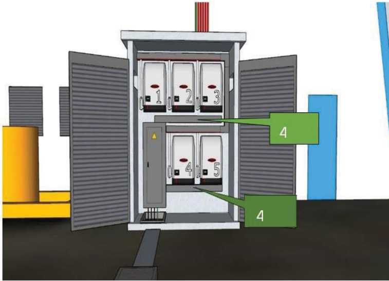
Figura. 6. Diseño en isométrico del gabinete para la instalación del centro de mando y control universal del sistema.
