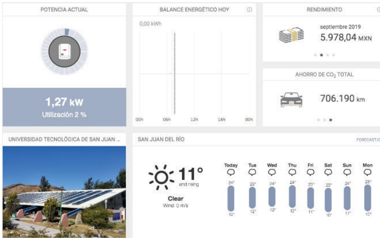
Figura 7. Datos obtenidos en tiempo real del comportamiento de la instalación fotovoltaica en el edificio “K” en la Universidad Tecnológica de San Juan del Río Fuente: https://www.solarweb.com/Home/GuestLogOn?pvSystemid=3752014d-7bdb-4867-b995-2d5foee9422f .
