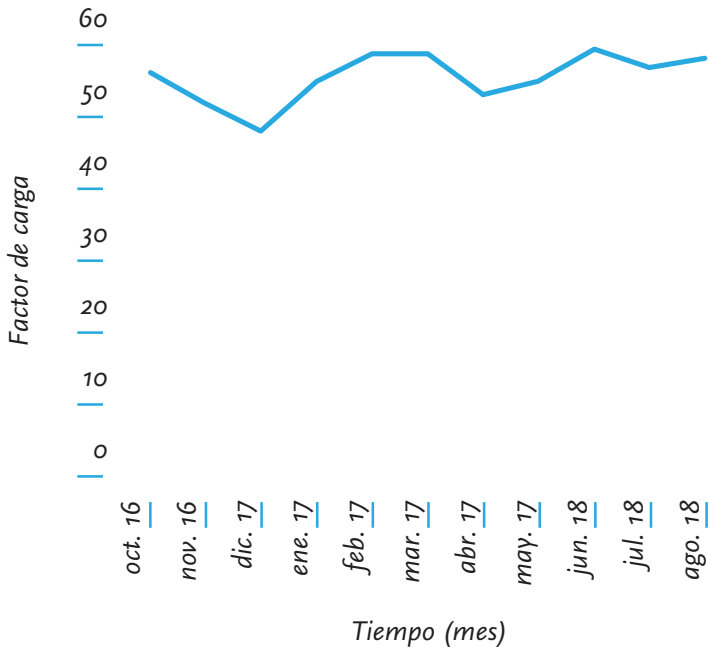
Gráfica 4. Análisis del comportamiento de la relación tiempo-factor de carga, en el edificio “K” en la Universidad Tecnológica de San Juan del Río.
