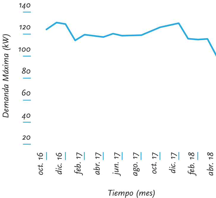
Gráfica 1. Análisis del comportamiento de la relación tiempo-demanda máxima, en el edificio “K” en la Universidad Tecnológica de San Juan del Río.
